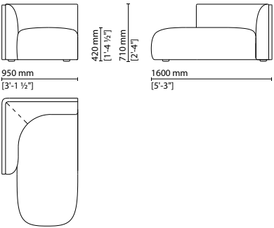
110 008 — Left Chaise Longue
