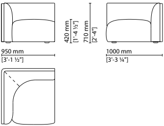
110 003 — Left End Unit
